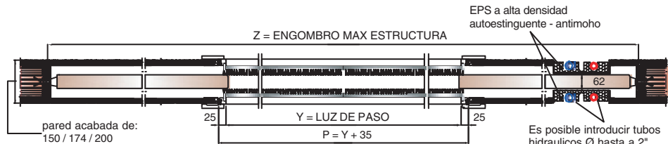
PANEL PUERTA
