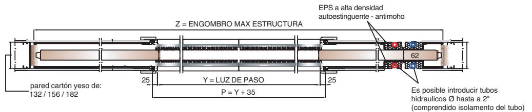
PANEL PUERTA
