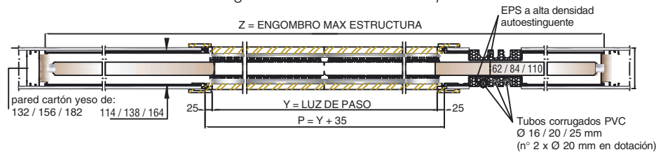
PANEL PUERTA
