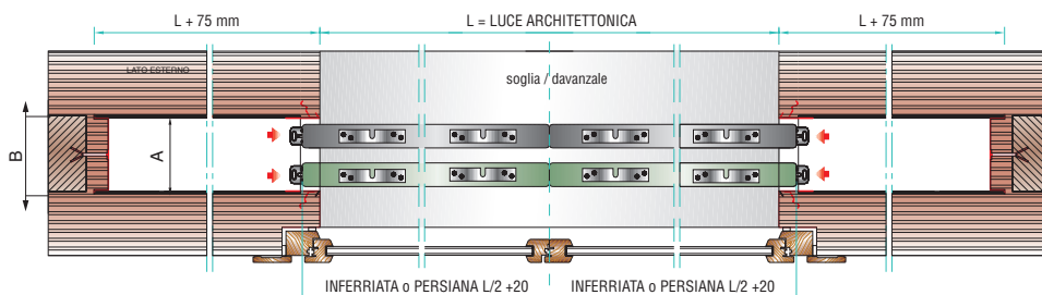
INFERRIATA O PERSIANA
